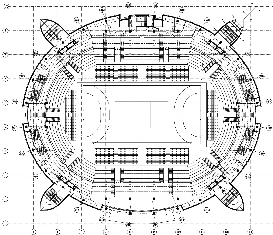
TLOCRT
