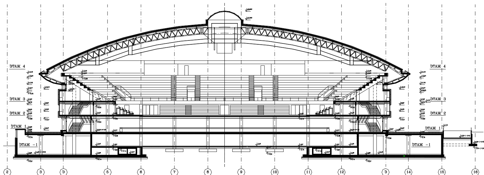
UZDUŽNI PRESJEK
